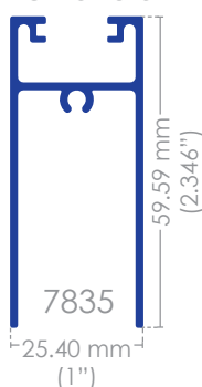
Zoclo ventana 3"
