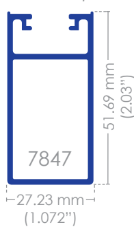
Cerco chapa 3"
