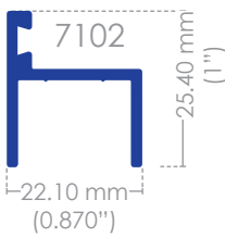
Batiente baño
