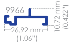
Adaptador mosquitero
