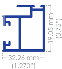
Traslape ventana 7844
