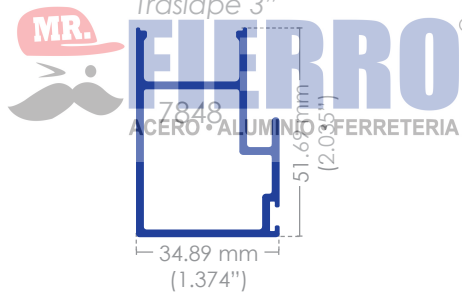
Traslape 3"
