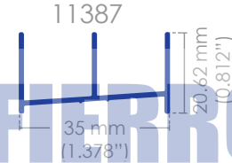
Riel vertical baño
