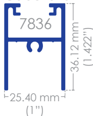
Cabezal 3"
