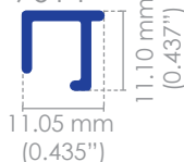
Junquillo 7014
