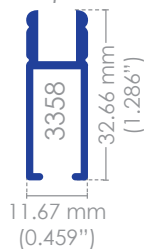
Zapata 3358
