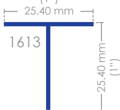
Tee ligera de 1"
